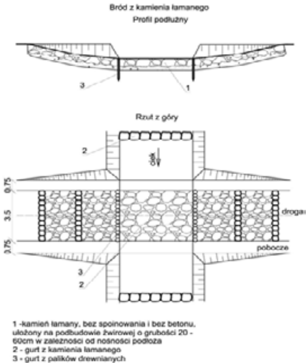
Rysunek 1.24 Bród z kamienia łamanego gr. 30 – 60 cm – RDLP w Krakowie Nadleśnictwo Łosie. Opracowano na podstawie: GDLP (2016)
