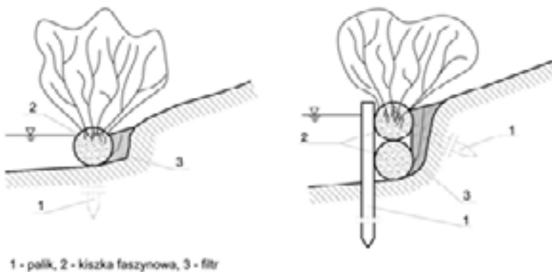
Rysunek 1.3 Opaska z kieszki faszynowej a) pojedynczej, b) podwójnej. Opracowano na podstawie: Żelazo, Popek (2014)
