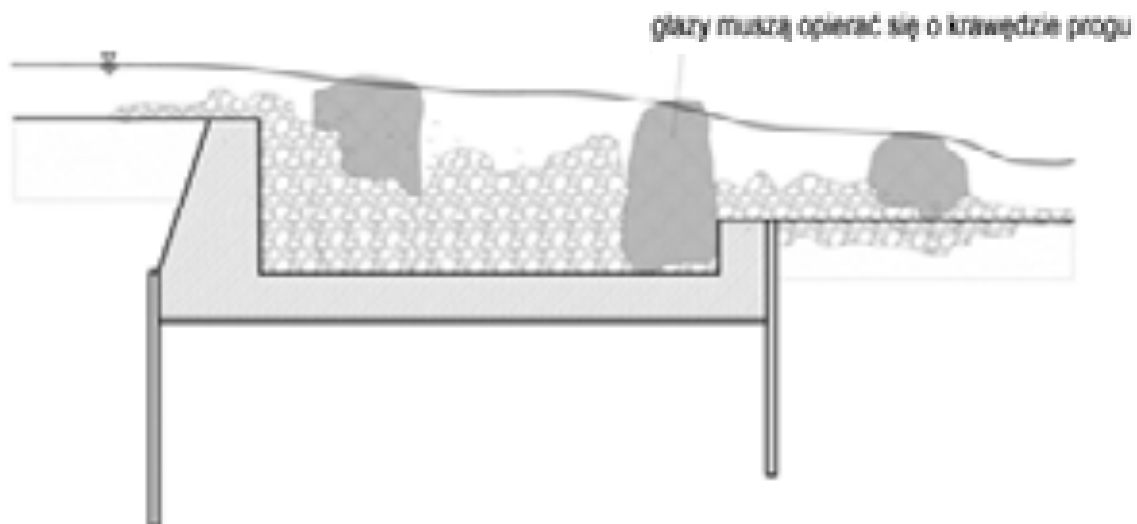
Rysunek 1.1 Przekształcenie jazu w pochylnię denną o szorstkim dnie. Opracowano na podstawie: Nawrocki (2016)
