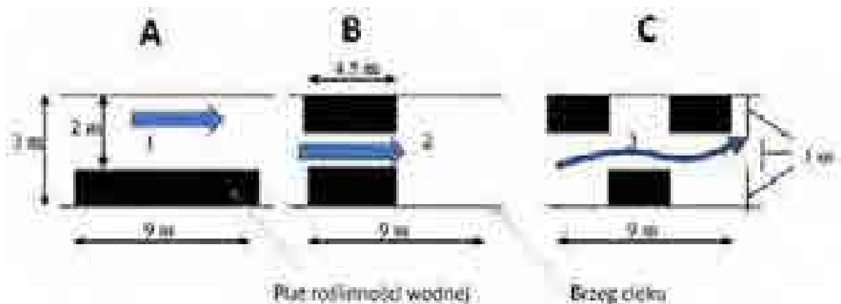
Rysunek 7.2 Rozmieszczenie roślinności porastającej dno cieku oraz występującej przy danej kompozycji roślinności kierunki przepływu wody (za Bal i in., 2011, zmienione). A – wykaszanie roślinności przy jednym brzegu rzeki, B -wykaszanie roślinności w środkowej części koryta, C – azurowe wykaszanie roślinności w korycie, naprzemiennie przy dwóch brzegach rzeki, będące najlepszą praktyką zarządzania roślinnością porastającą dna cieków.
