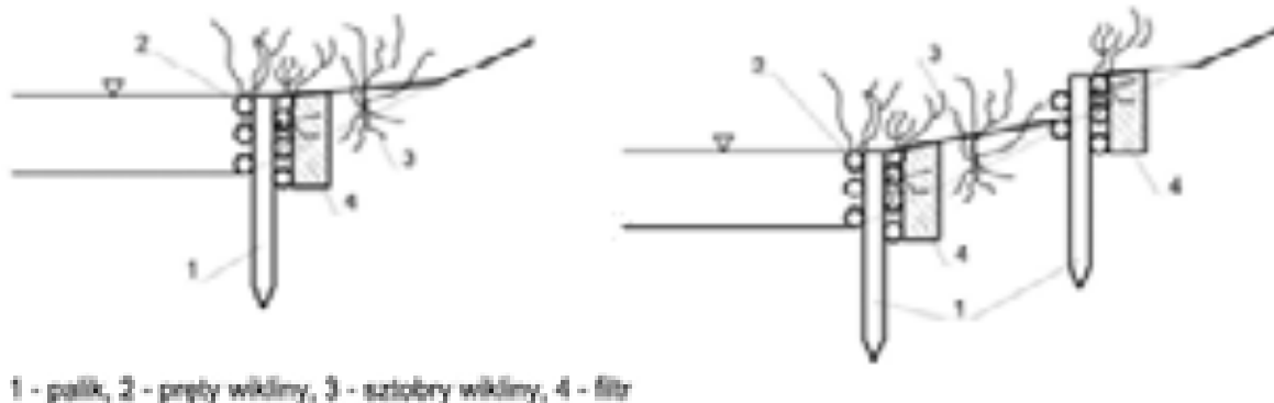
Rysunek 1.2 Opaska z plotka faszynowego. Opracowano na podstawie: Żelazo, Popek (2014)
