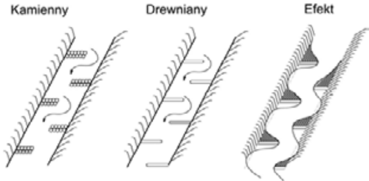
Rysunek 1.11 Naprzemienne rozmieszczenie deflektorów/ostrog z materiałów naturalnych. Opracowano na podstawie: GDLP (2016)
