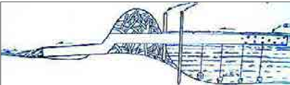
Rysunek 7.4 Schematy umieszczania rur w tamach bobrowych. Źródło: www.bobry.org
