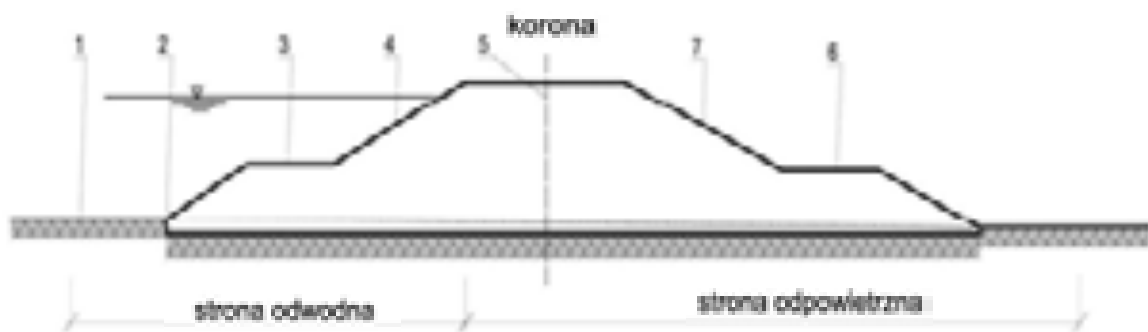
1 - międzywał, 2 - stopa skarpy odwodnej, 3 - laweczka odwodna, 4 - skarpa odwodna, 5 - oś wału, 6 - laweczka odpowietrzna, 7 - skarpa odpowietrzna
