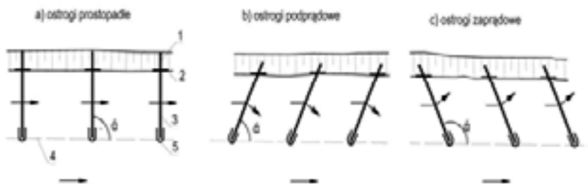
1 - wrzynka, 2 - opaska, 3 - korpus, 4 - linia regulacyjna, 5 - głowica
