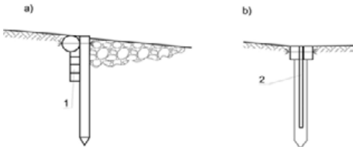
Rysunek 1.19 a) gurt z jednego lub dwóch okrągłaków i ścianki szczelnej, b) gurt ze ścianki szczelnej pojedynczej. Opracowano na podstawie: Wołoszyn, Czamara, Eliasiewicz, Krężel (1994)
