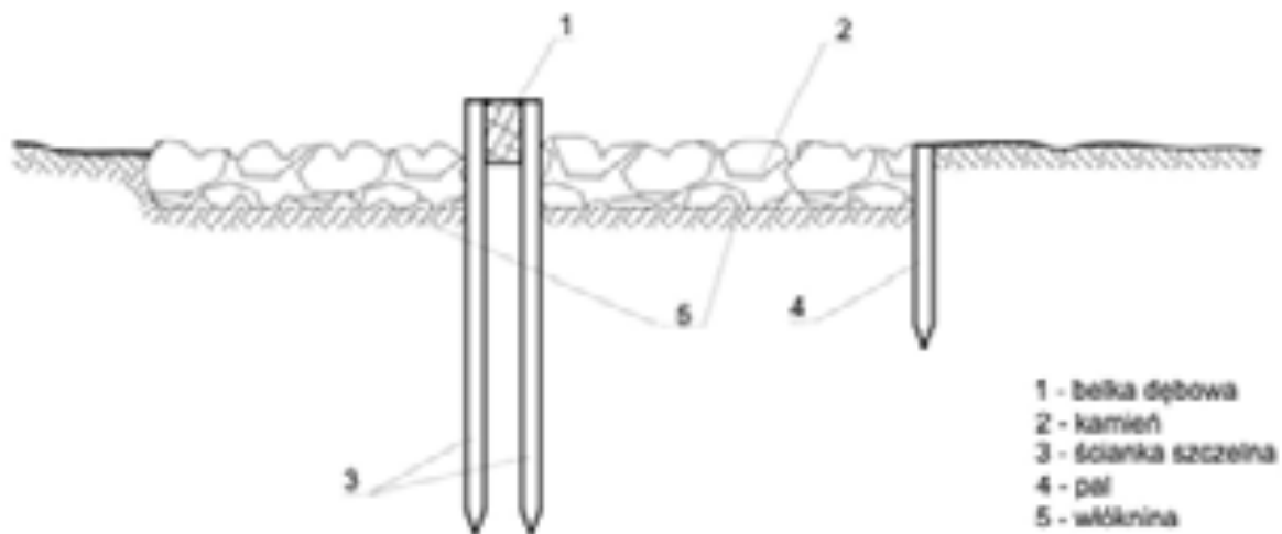
Rysunek 1.20 Próóg drewniany z wypadem kamiennym. Opracowano na podstawie: Jędryka (2006)
