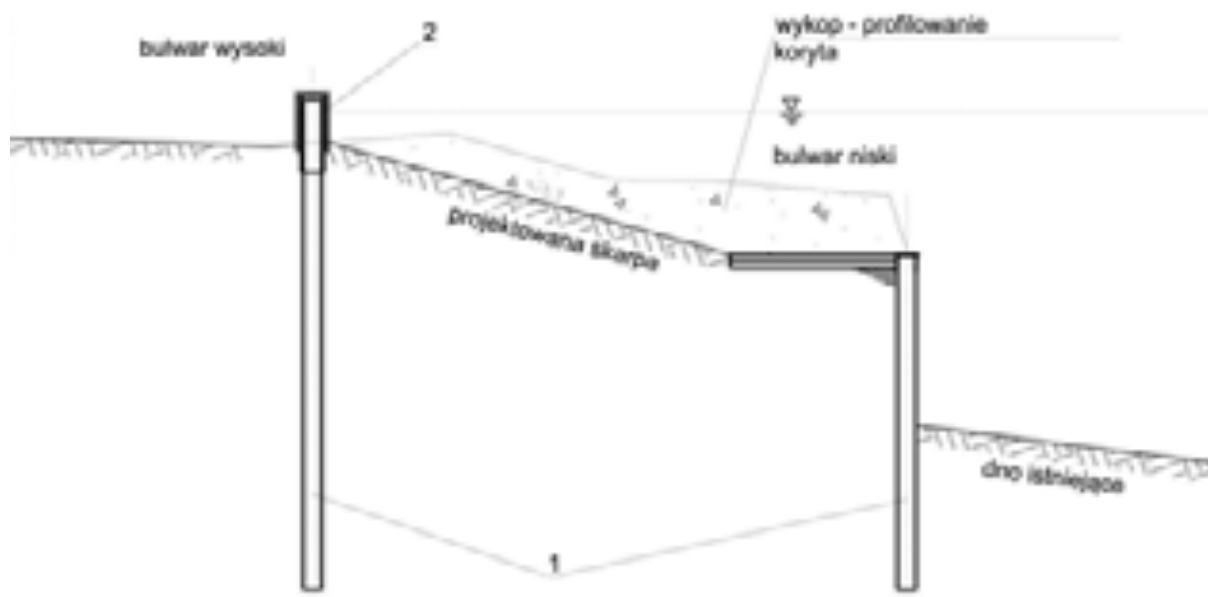
1 - stalowa ścianka szczelna, 2 -ociep belbełowy
