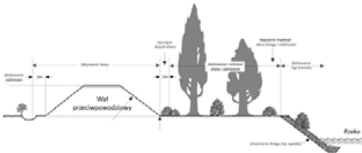
Rysunek 7.3 Przykład dobrych praktyk zarządzania roślinnością w międzywalu. Opracowano na podstawie: BC Ministry of Environment, 1999, zmienione
