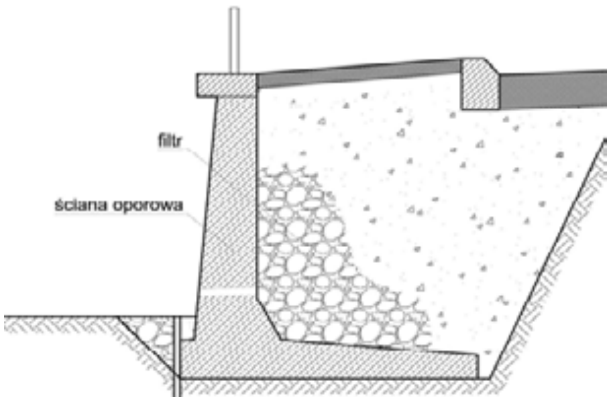
Rysunek 1.8 Ściana oporowa, żelbetowa. Opracowano na podstawie: Wołoszyn, Czamara, Eliasiewicz, Krężel (1994)
